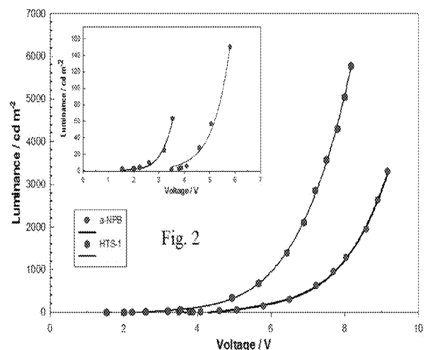
1-萘基-9-基-噻吩，1-联苯-4-基-噻吩和9，10-双（1-噻吩基）蒽。
