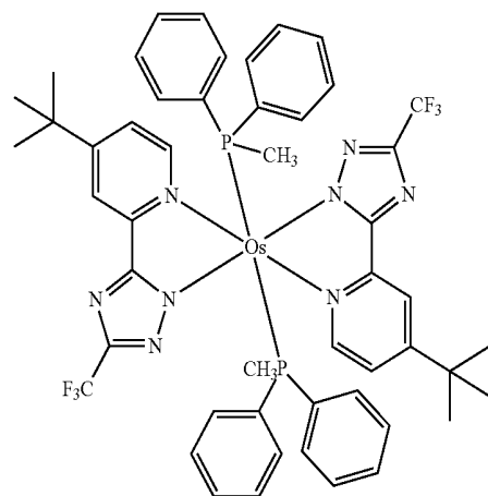
Os(bpftz) 2 (PPh 2 Me) 2
